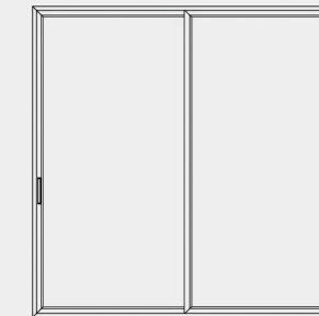
V350 Sliding Door
